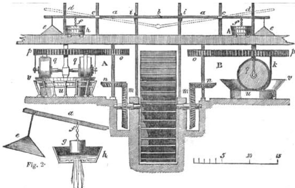
Figuren over viser et vanddrevet anlegg fra slutten av 1700-tallet. Det spesielle med denne konstruksjonen er at den har et automatisk brannslukkeanlegg plassert over møllene (fig. 2).
