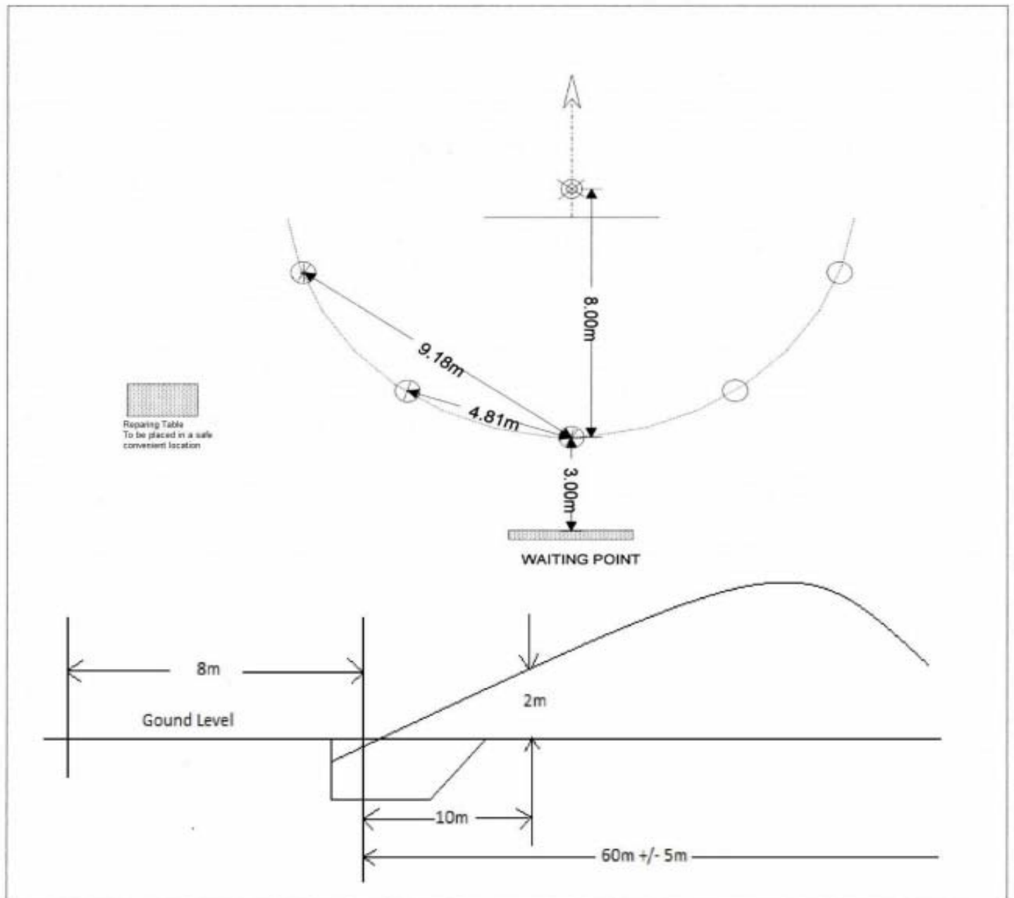
Prinsippskisse av haglebane
